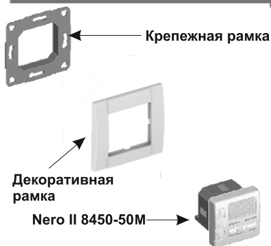
Рисунок 1. Установка устройства
